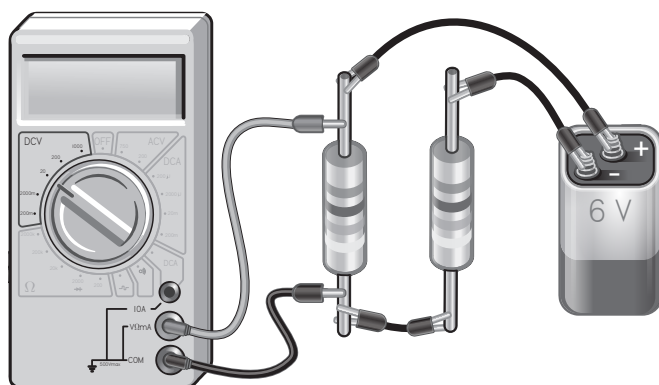
a) Mesure d'un courant compris entre 200 mA et 10 A.
