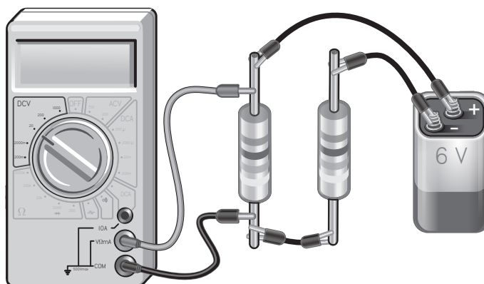
Mesure d'une tension continue
