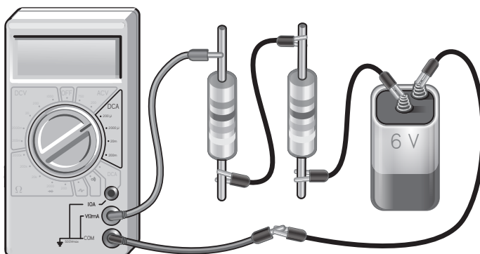
Mesure d'un courant inférieur à 200 mA
